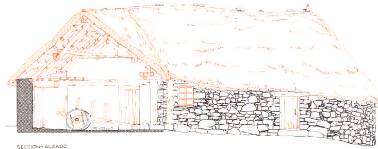
Sección de una palloza. Arquitectura Popular Leonesa. J.L. García Grinda.
